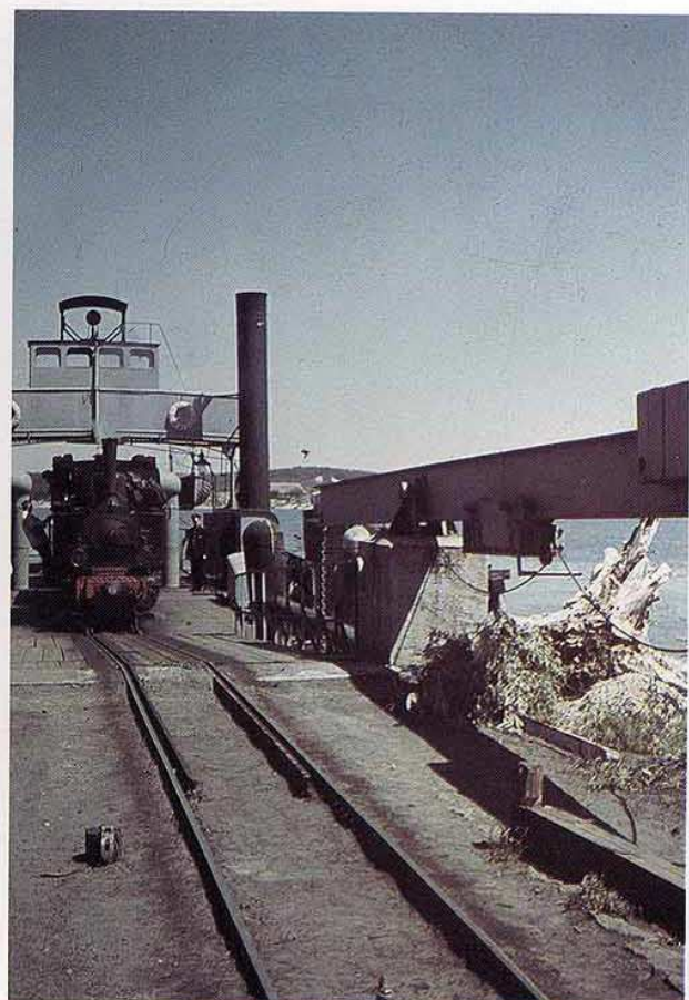
Weichselfähre mit Lok am Durchstich Nickelwalde-Schiewenhorst, um 1940. (Farbe 11/2)
