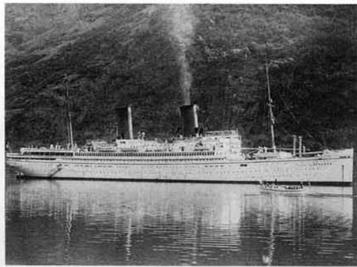
General von Steuben, Baujahr 1922, 14660 BRT, Nordd. Lloyd, Bremen. Versenkt am 10.2.1945, 3000 Tote. (Fluchtschiff 5)
